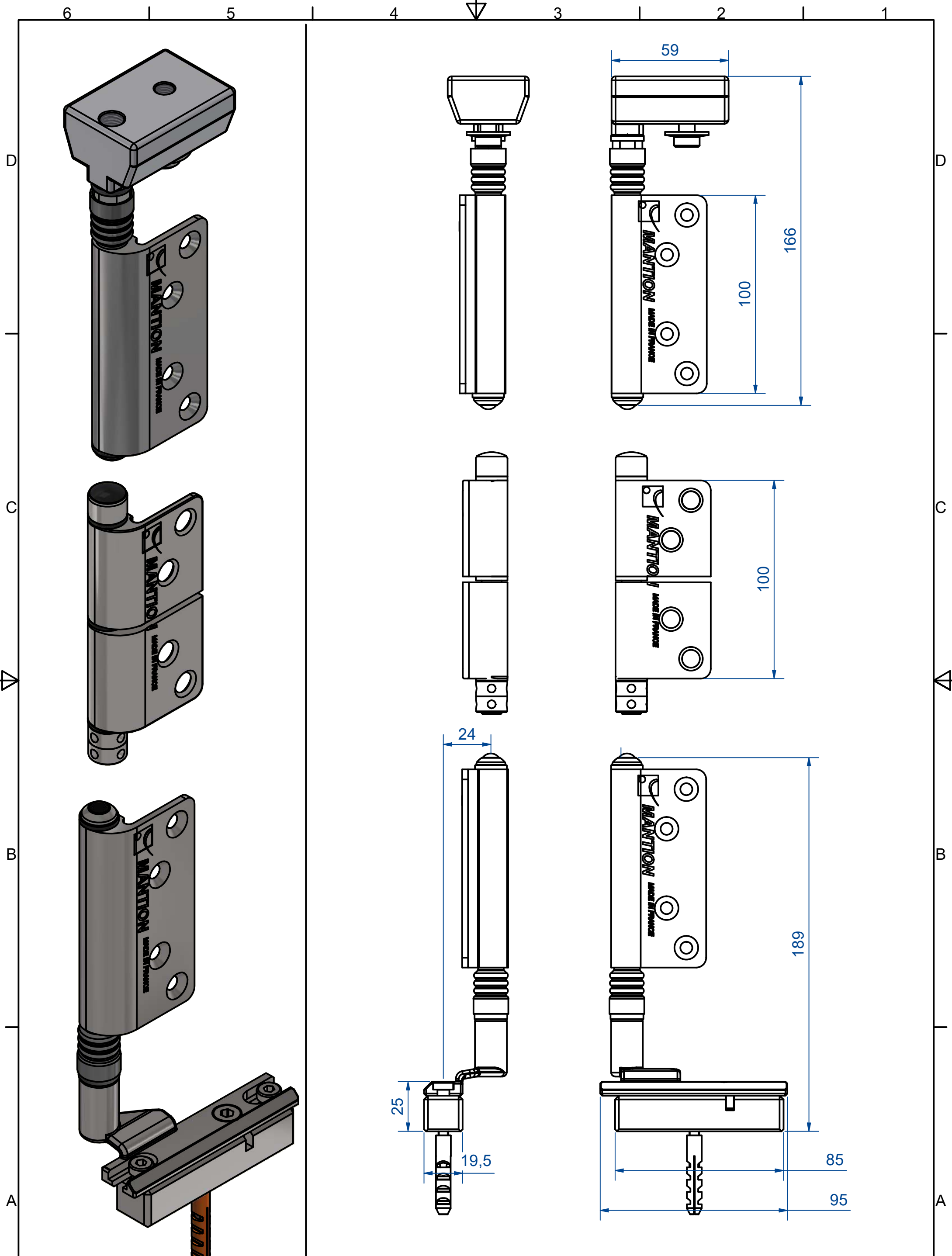
Set point fixe gauche FWF100 Set left pivot assembly FWF100
