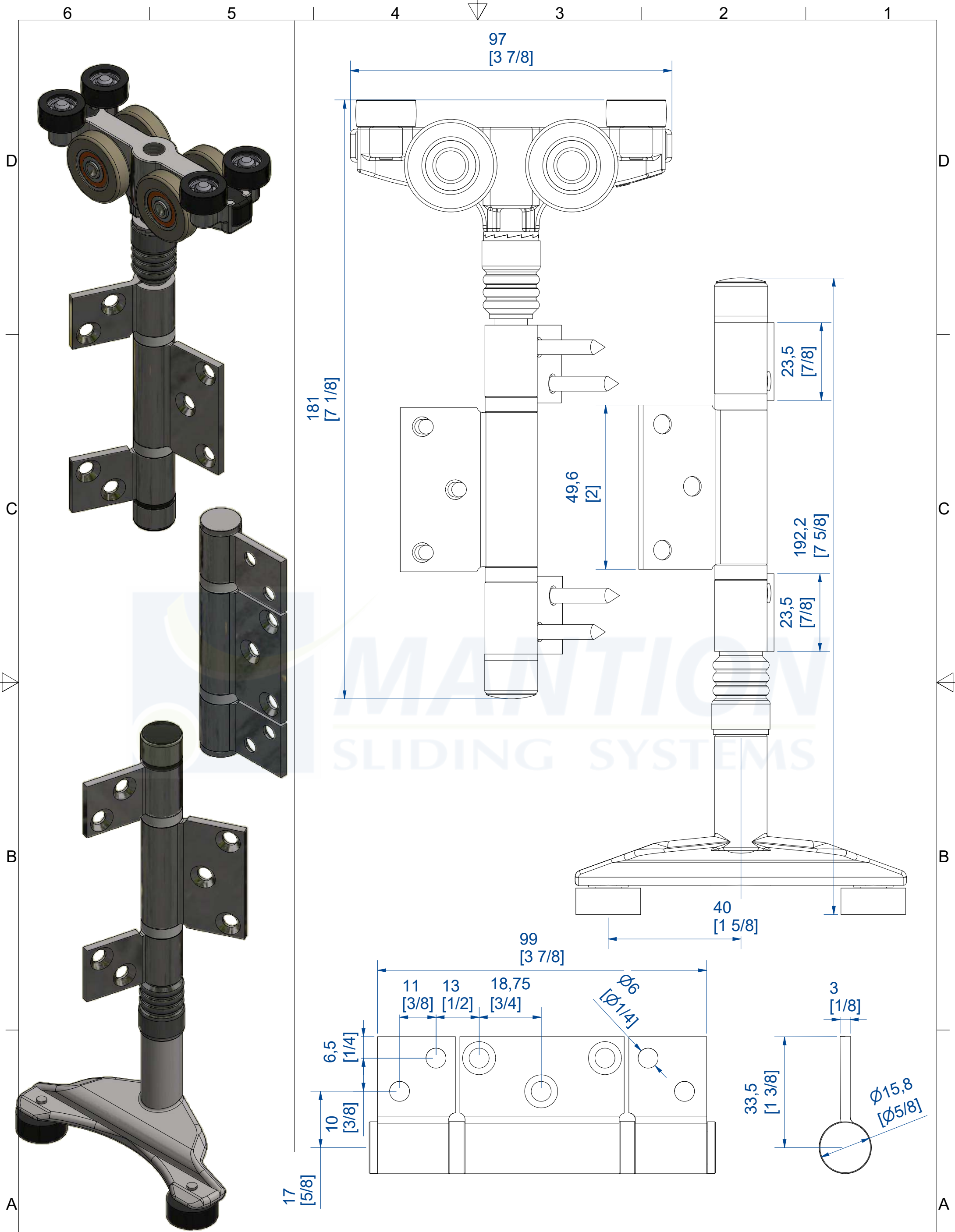
Set montage intermédiaire FWF100 Set intermediate hanger FWF100
