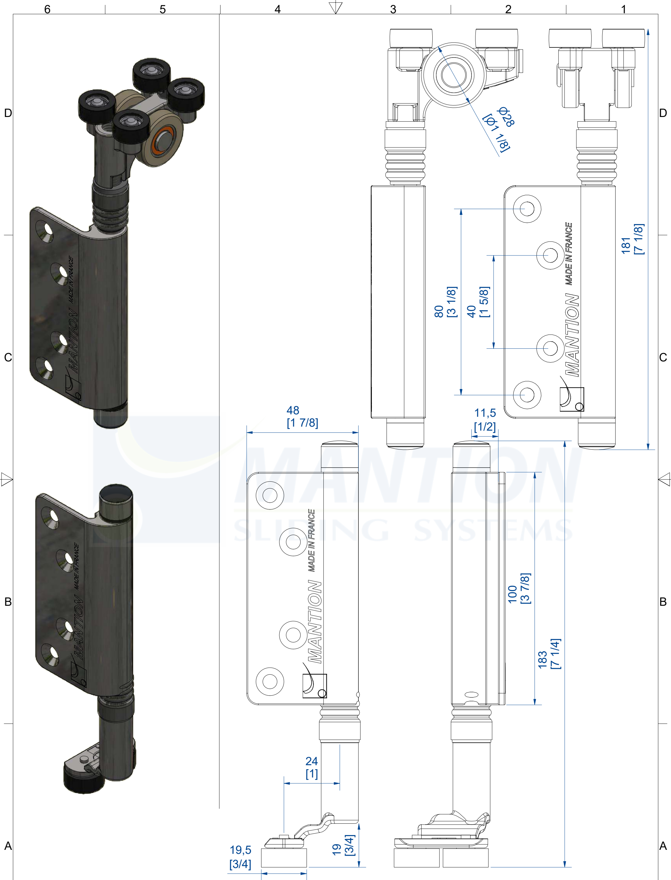
Set monture extrémité droit FWF100 Set right end hanger FWF100
