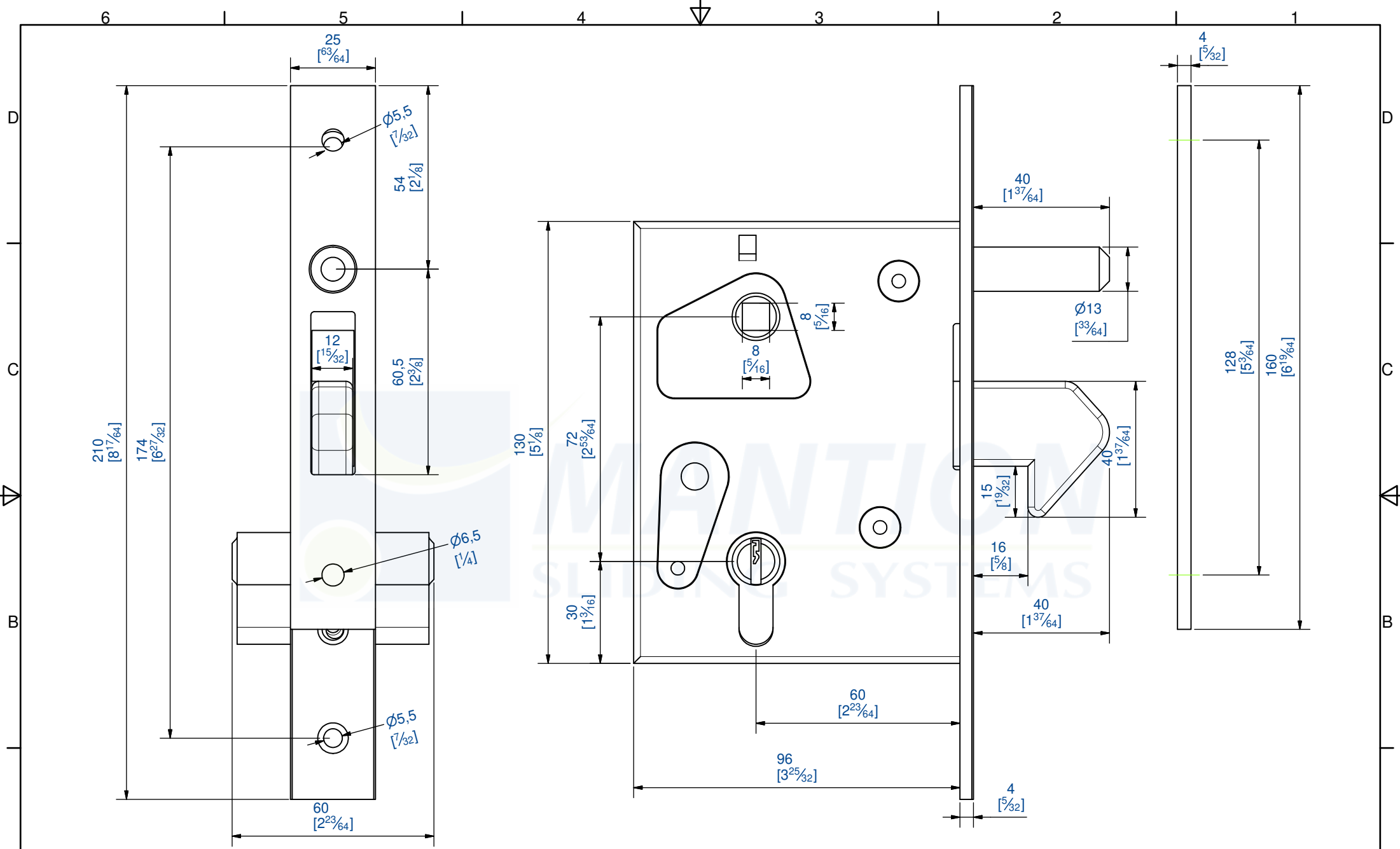
A Serrure à crochet galvanisée -Cylindre européen & 3 clés Hook lock in galvanised steel - European Cylinder and 3 keys
