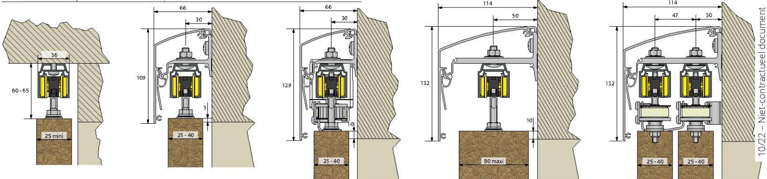
Plafondbevestiging Muurbevestiging eenwegs Muurbevestiging eenwegs gemotoriseerd Muurbevestiging (zonnescerm) Muurbevestiging tweewegs gesynchroniseerd
