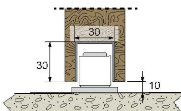
Guide 1081 + profile 1110
