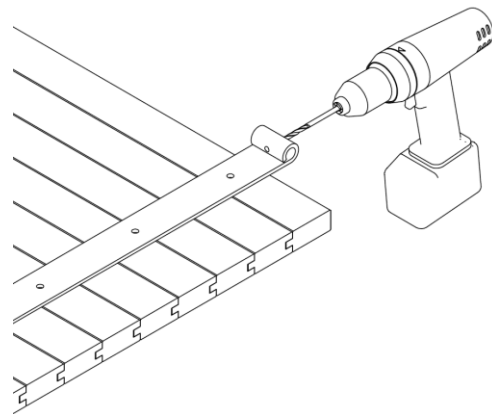
Perçage parallèle
