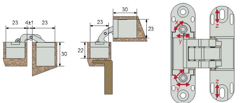
Charnière 1540 encombrement réduit
