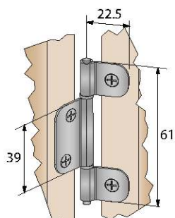
Charnière sur chant 1504C3
