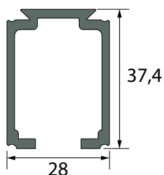
Rail 11312/... (2 - 3 - 5 - 6 m)
