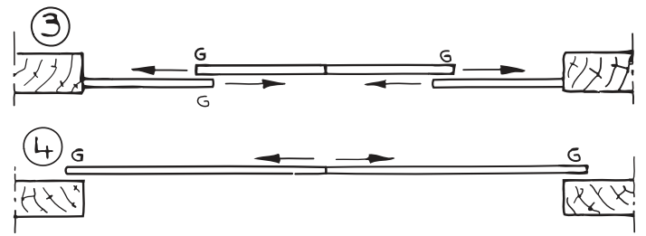
Fig. 7 : Exemples de portes réalisables avec le patin MINITUB.
