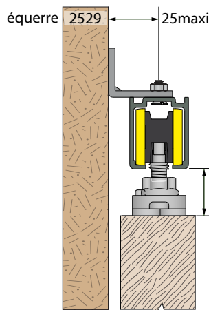
Montage fixation murale avec équerre 2529 (MA80)
