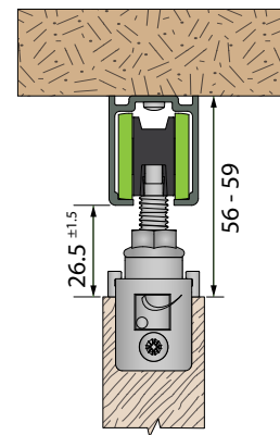
Montage fixation plafond avec platine 11036L
