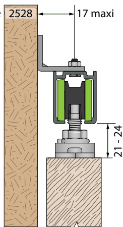
Montage fixation murale avec équerre 2528 (MA40)
