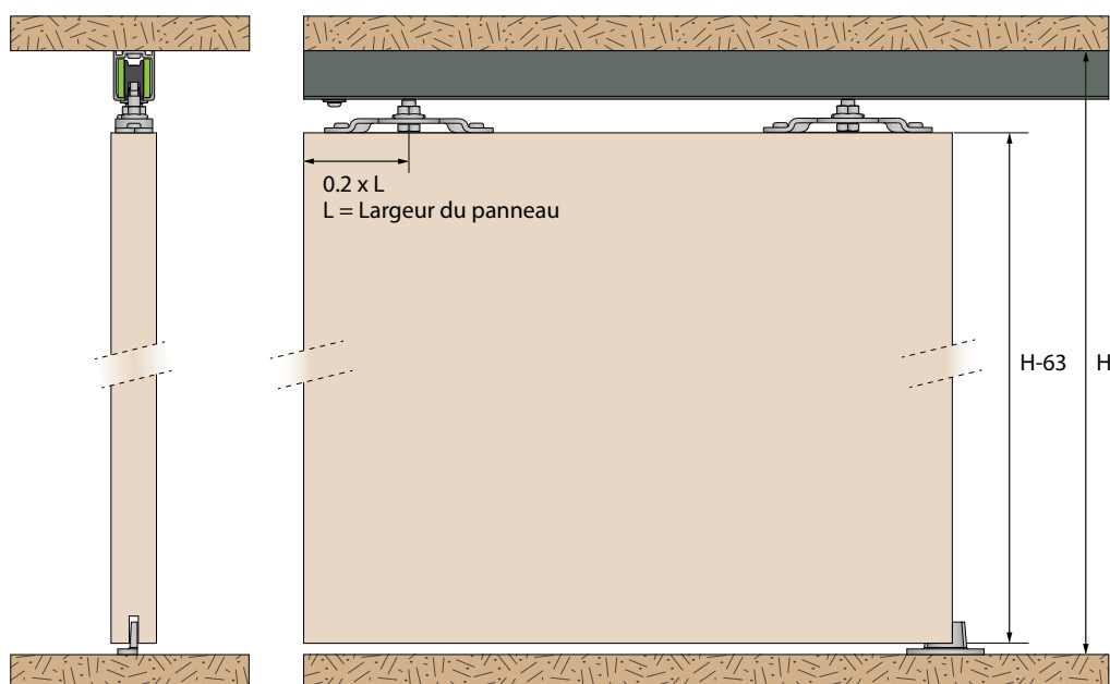
Montage guide 1103 avec profil 1106
