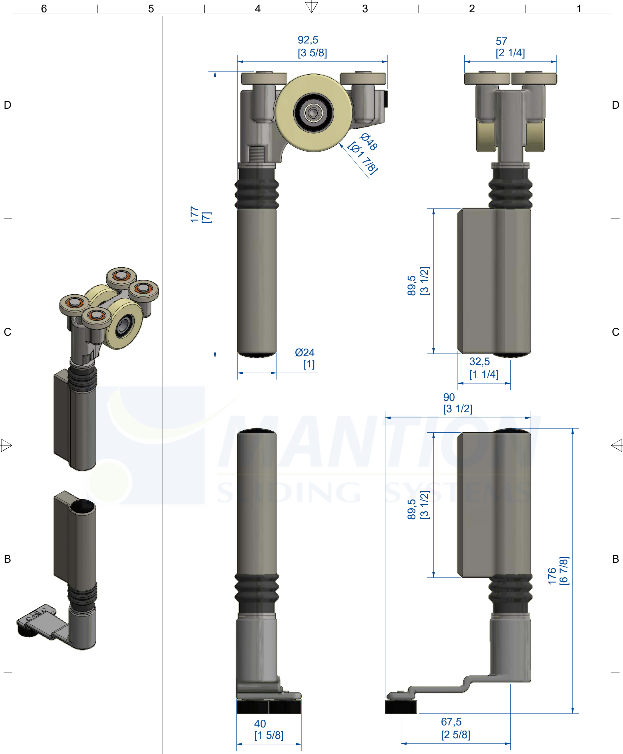
Set monture d'extrémité gauche FMF150
