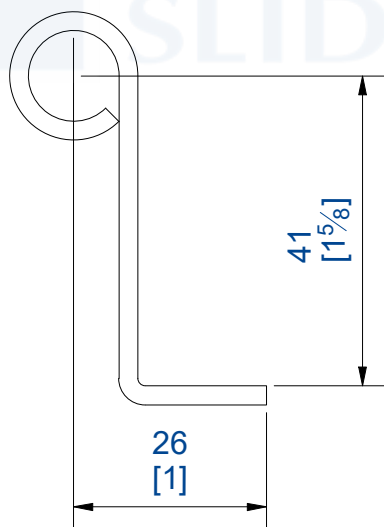
Guide du bas d'extrémité déporté pour U 30x30. (1110)
