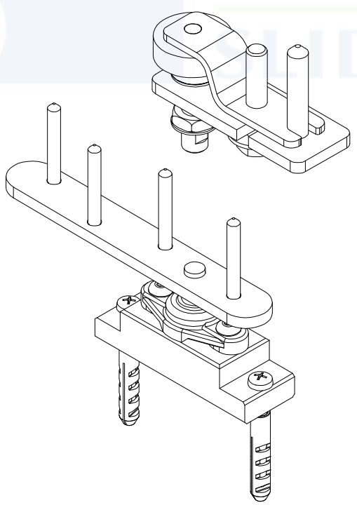
PIVOT HAUT + BAS PLIANT OPENTEC FW75 TOP + BOTTOM PIVOTS FOLDING OPENTEC FW75
