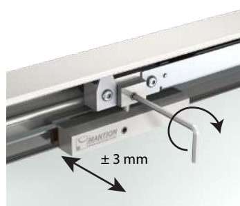
Montage fixation plafond Réglage en profondeur avec paroi fixe
