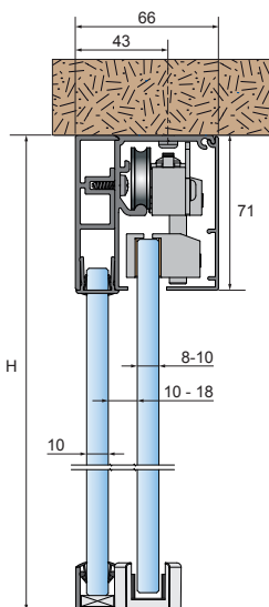
Montage fixation plafond Réglage en profondeur avec paroi fixe
