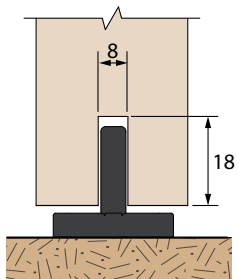
Montage guide 1103R
