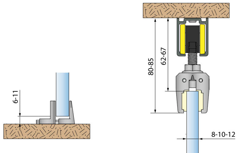
Montage avec guide 1124
