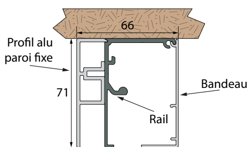
Rail fixation plafond avec paroi fixe
