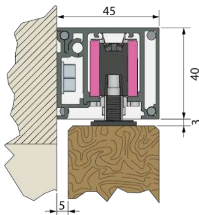
Montage fixation murale
