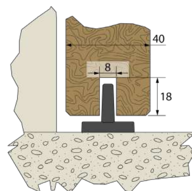
Montage guide 1103R
