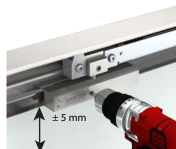
Réglage en hauteur
