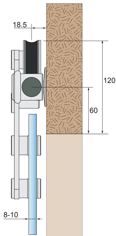
Montage fixation murale
