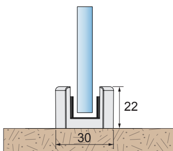
Montage guide 1112/4
