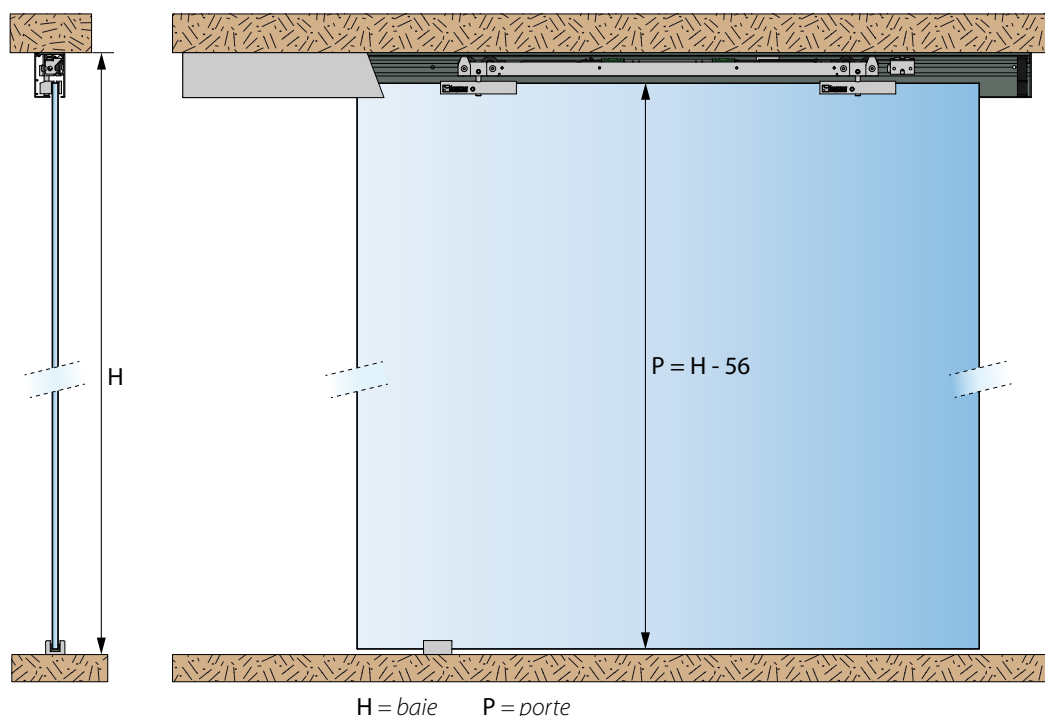
Rail fixation plafond + bandeau
