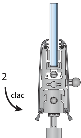
Clipsage des bandeaux
