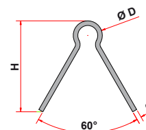
RAIL À SCELLER POUR GORGE RONDE acier galvanisé - barres de 3 Mètres 20021RS/3 D = 19 / e = 3 / H = 60
